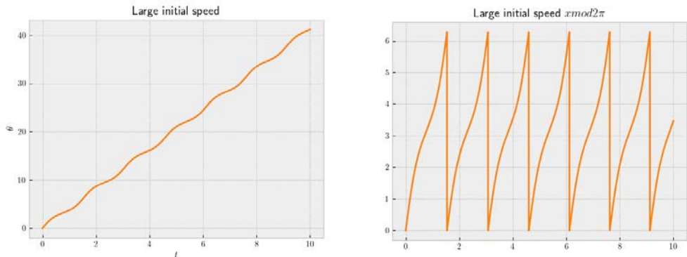
Εικόνα 5. Διάγραμμα \theta - t για την προσομοίωση (γ)
