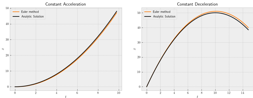
Εικόνα 2. Διαγράμματα Σύγκρισης Προσομοίωσης (πορτοκαλί) και Θεωρίας (μαύρο).
